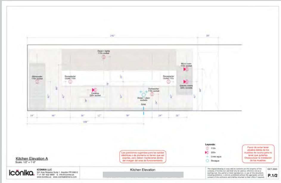
Ejemplo de Plano de Elevación de Utilidades y Dimensiones
