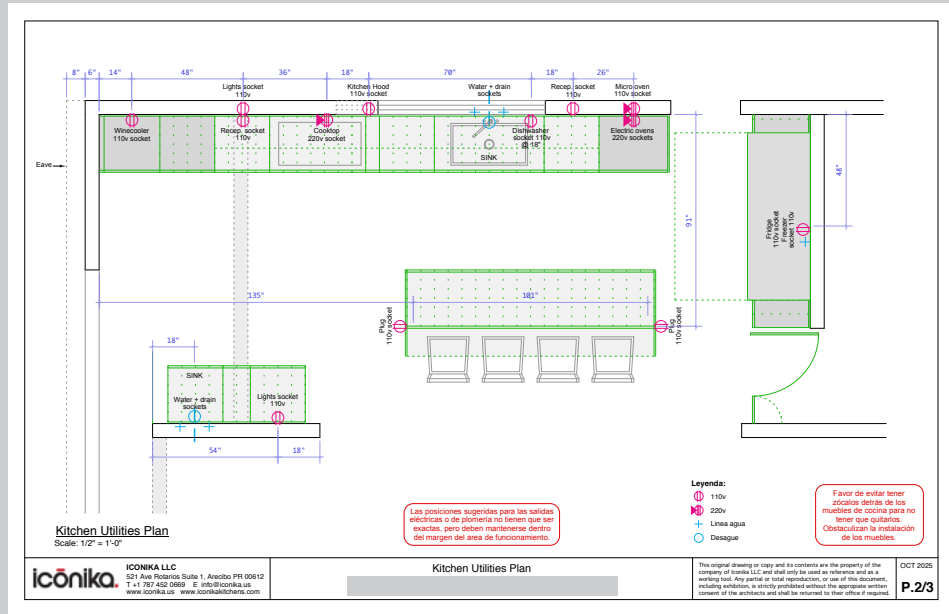
Ejemplo de Plano en Planta de Utilidades y Dimensiones
